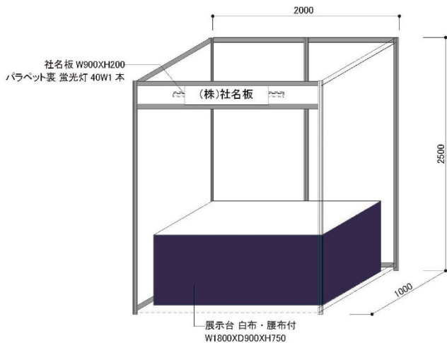
— 小間規格:A、Cタイプ共通 —
